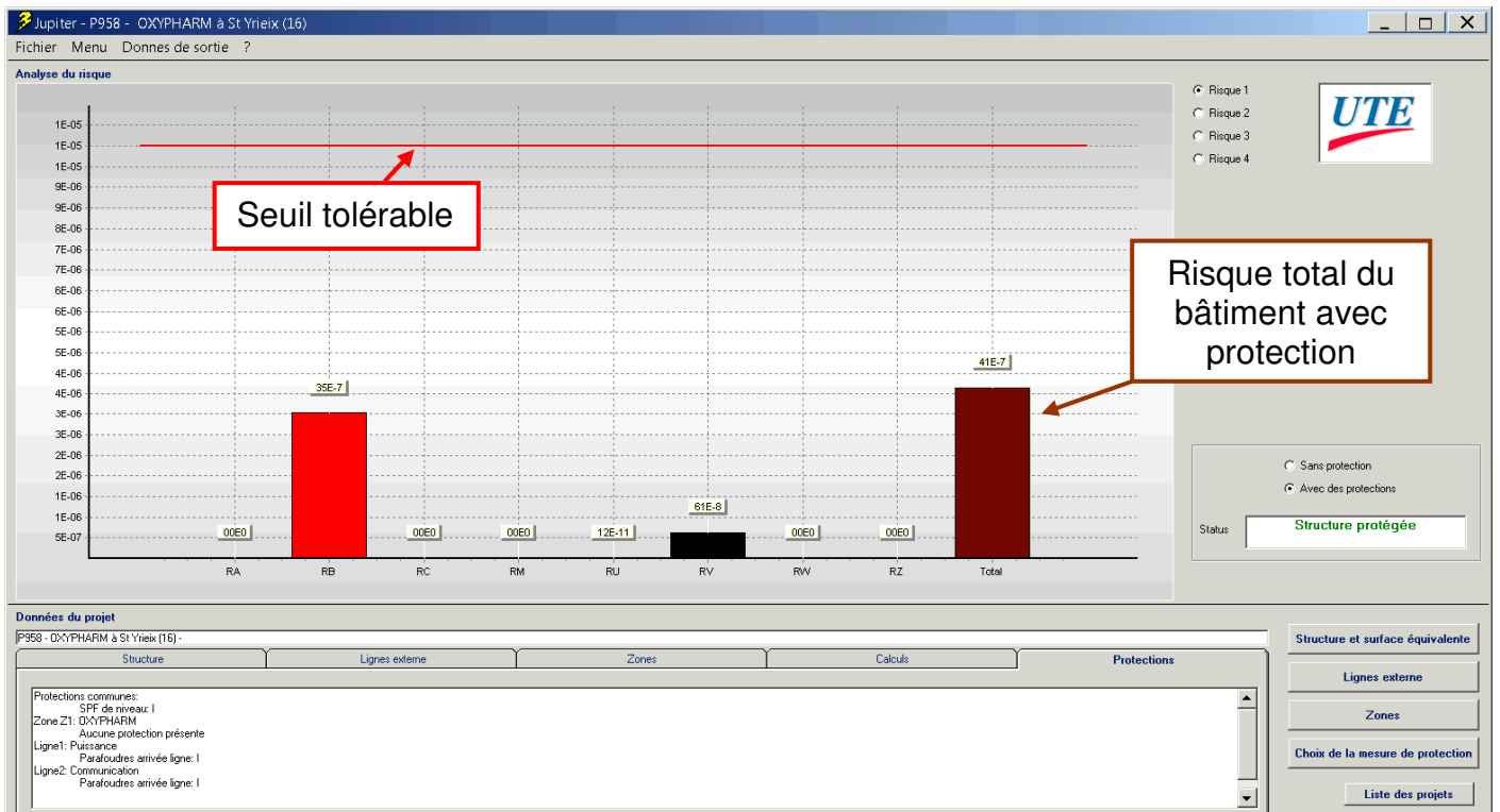
Résultat de l'Analyse de Risque Foudre : Avec protection de niveau I
